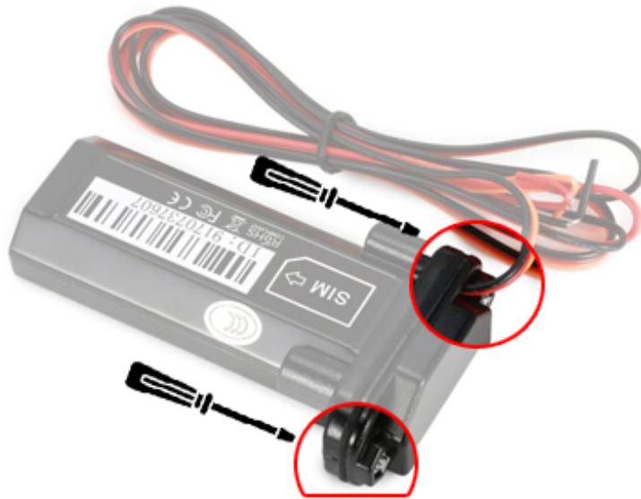
Abb. 3 Lösen der Schrauben
