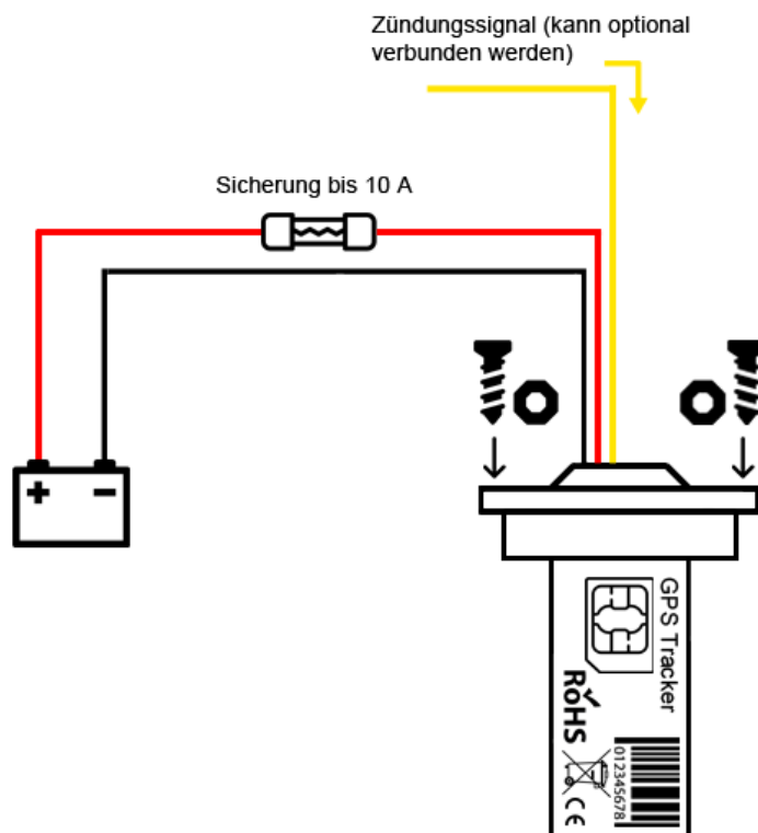
Abb. 6 Schematische Darstellung der Beschaltung des GPS Ortungsgeräts
